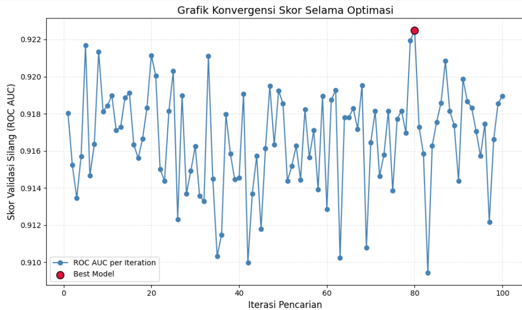
Gambar 4.25 Grafik Konvergensi Skor Selama Optimasi
