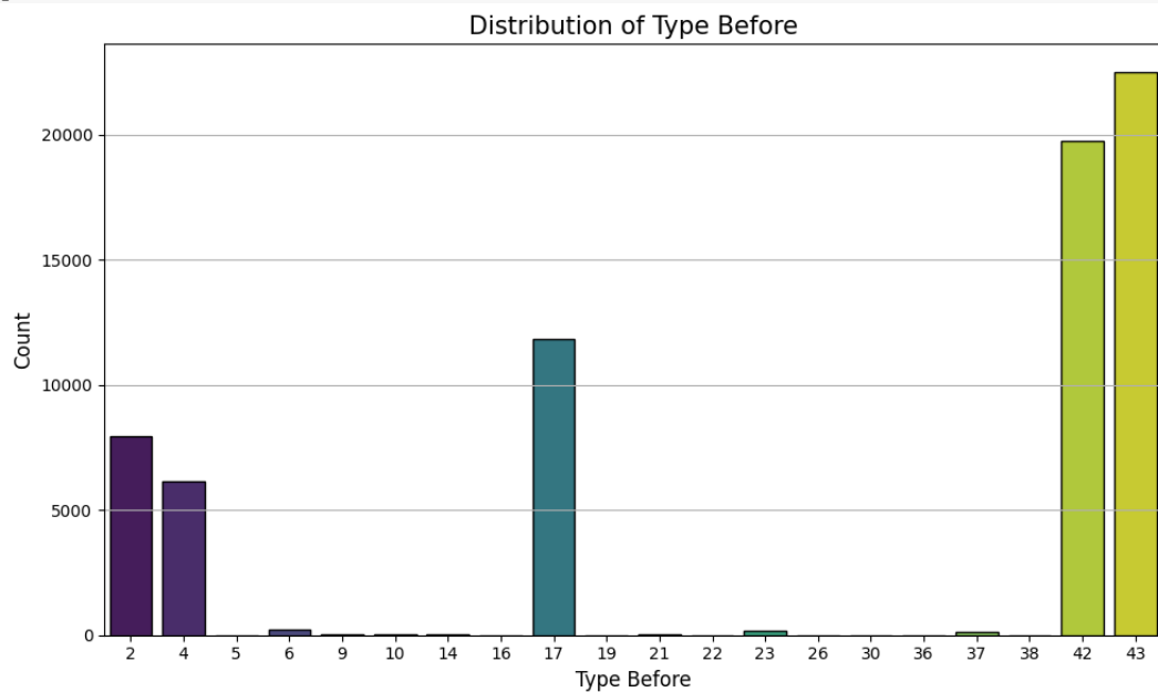
Gambar 4.24 Distribusi Jenis Peristiwa Sebelum Tembakan ( Type Before )
