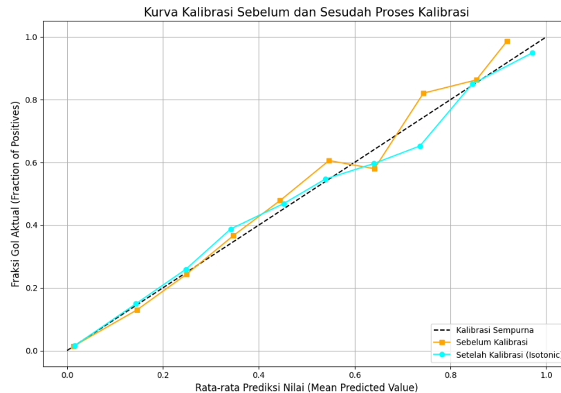
Gambar 4.27 Kurva Kalibrasi Sebelum dan Sesudah Proses Kalibrasi
