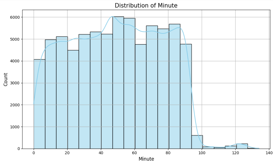
Gambar 4.8 Distribusi Menit Pertandingan
