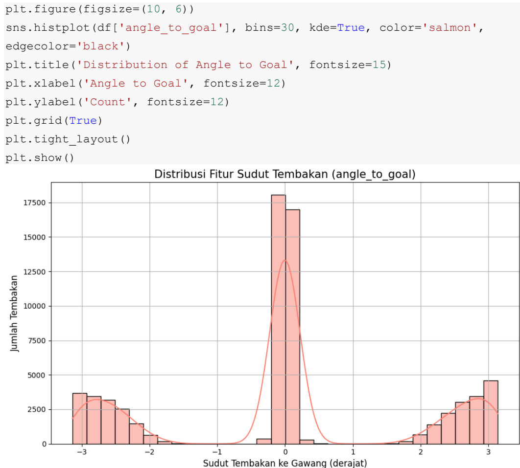
Gambar 4.23 Visualisasi Distribusi Fitur angle_to_goal
