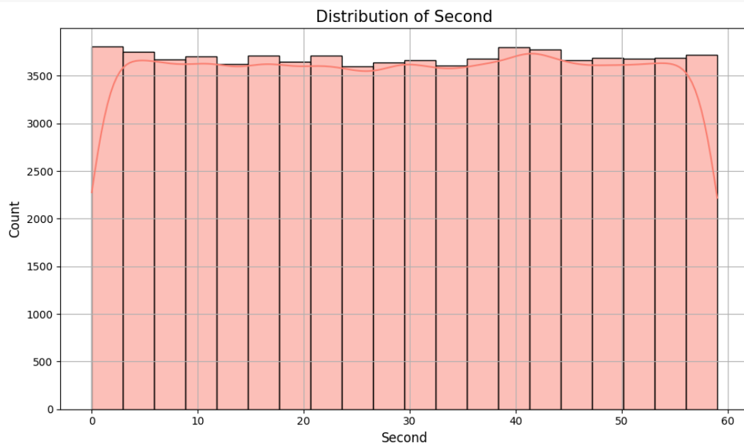
Gambar 4.9 Distribusi Detik Pertandingan
