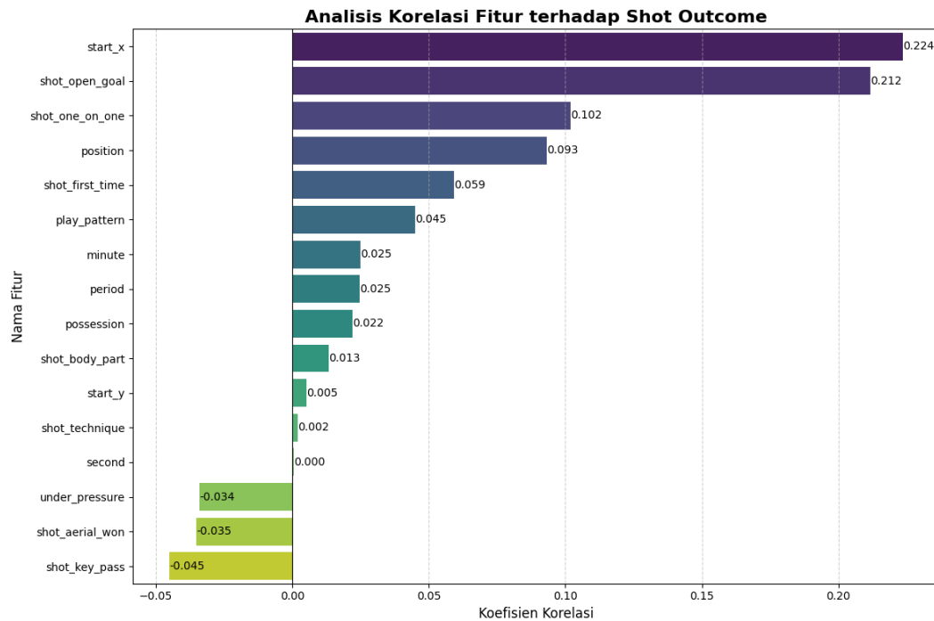
Gambar 4.18 Analisis Korelasi Fitur
